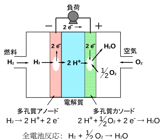
燃料電池の作動原理
